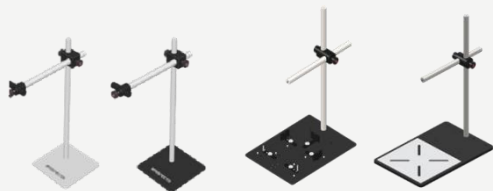
HD-060-EXT, Штатив с одной штангой, 500мм LWD HD-060-E-EXT, Штатив с одной штангой, 500мм LWD, ESD HD-060-LWD-LB-E, Штатив с одной штангой, LWD с держателем платы, ESD HD-060-LWD-HD-E, Штатив с одной штангой, LWD, усил. основание, ESD.
